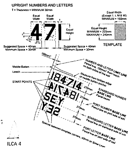
ILCA4 帆示意图
