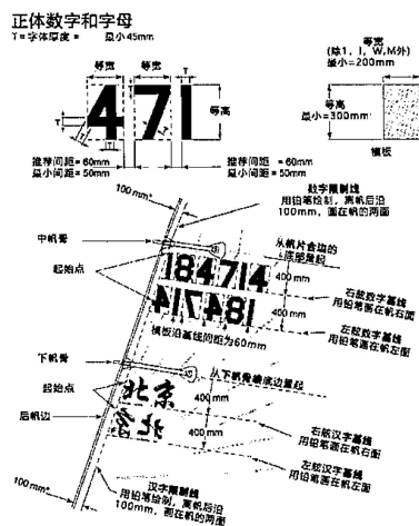
ILCA6 帆示意图
